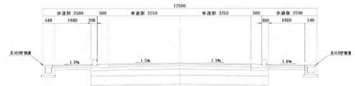
標準横断面
